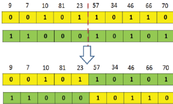
Fig. 6. Crossover step.
