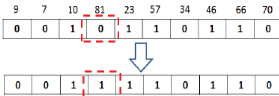
Fig. 7. Mutation step.
